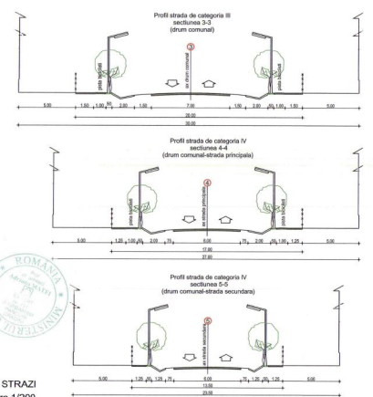
PROFILI STRAZI scara 1/200
